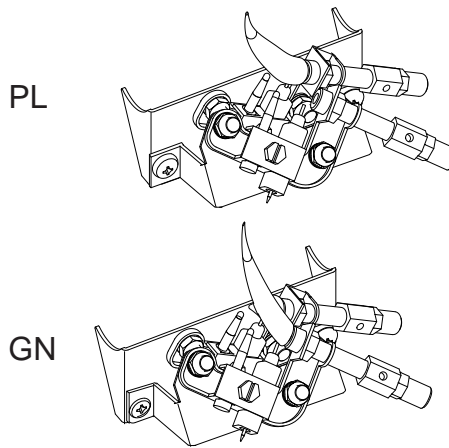
Fig. 27 - Patrón incorrecto de llama piloto
