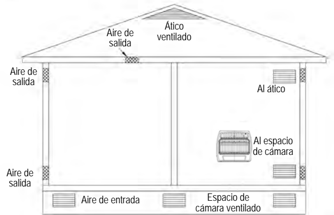
Fig. 2 - Aire de ventilación de aire libre
