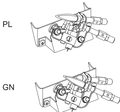
Fig. 26 - Patrón correcto de llama piloto
