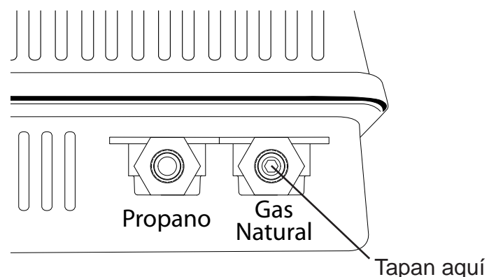
Fig. 6 - El ubicación de la clavija reguladora
