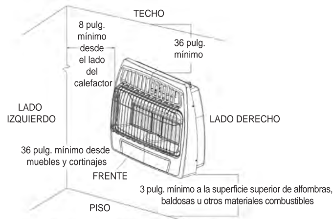
Fig. 2 - Espacios libres de montaje vistos desde el frente del calefactor (pulgadas)
